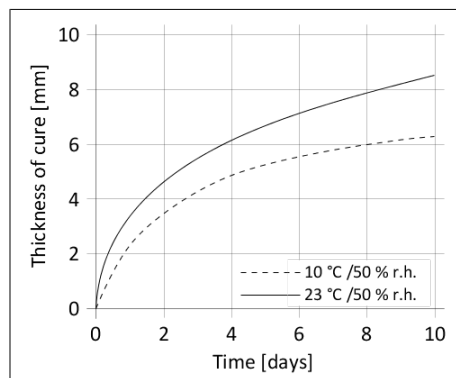
Diagrama 1: Velocidad de curado de Sikaflex®-552 AT
