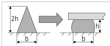
Figura 1: Configuración recomendada para el cordón
