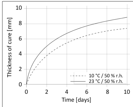
Diagrama 1: Velocidad de curado de Sikaflex®-292i
