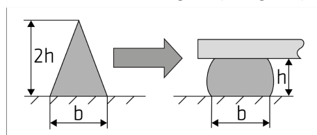
Figura 1: Configuración del cordón recomendado
