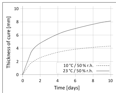
Diagrama 1: Velocidad de curado de Sikaflex®-552
